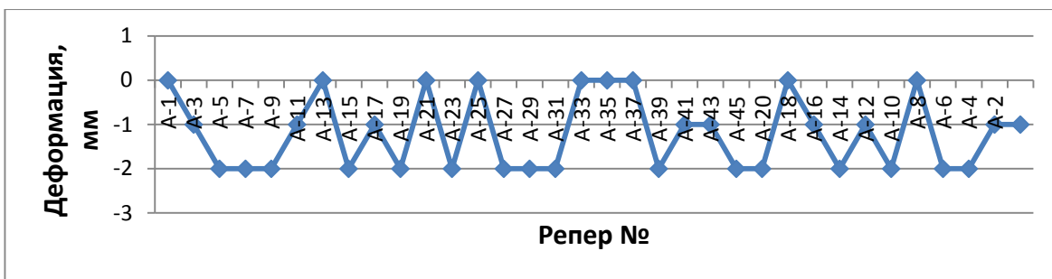
25 Сурет – «Мәскеу» бекеті аймағындағы 2014-2017 жылдар аралығындағы реперлер деформациясының графигі
