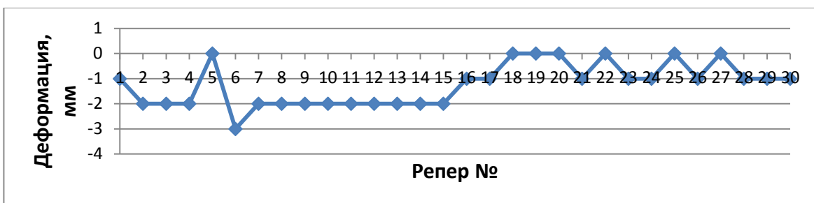
26 Сурет – «Сарыарка» бекеті аймағындағы 2014-2017 жылдар аралығындағы реперлер деформациясының графигі
