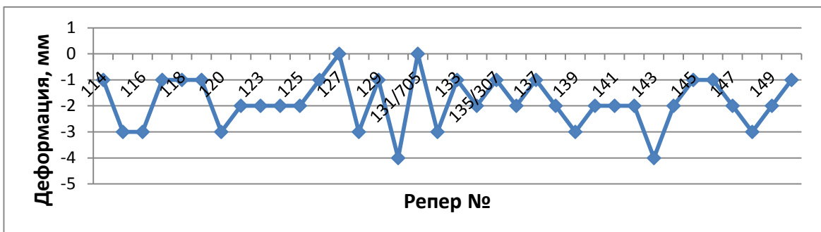
27 Сурет – «Достық» бекеті аймағындағы 2014-2017 жылдар аралығындағы реперлер деформациясының графигі
