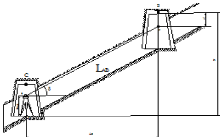
14 Сурет – Қазбаларға тригонометриялық бағыт беру сұлбасы
